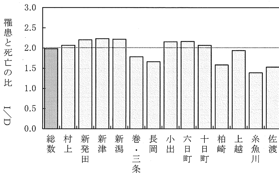
図3 地区別 I/D
