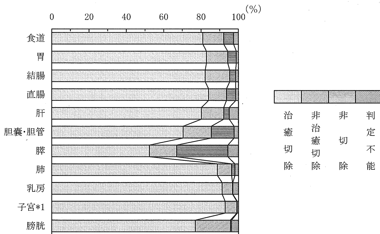
図10 手術の程度
