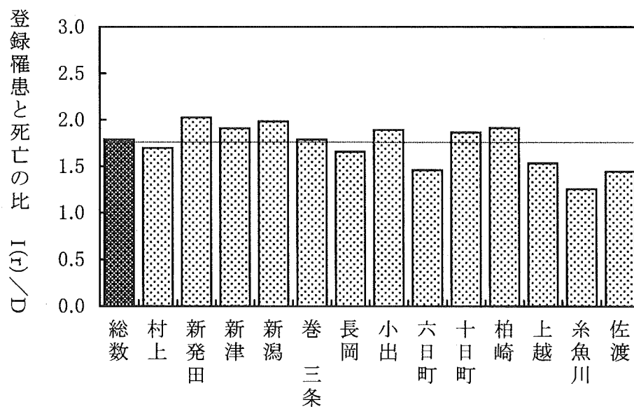
図3 地区別 I(r)/D
